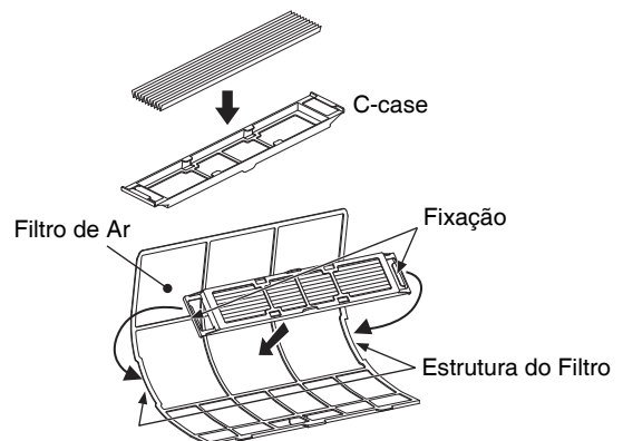
Malha de Limpeza de Ar Wasabi-Nano Titanium (Wasabi-Nano Titânio)
